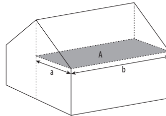
Anzuschließende Dachgrundfläche A = a \cdot b
